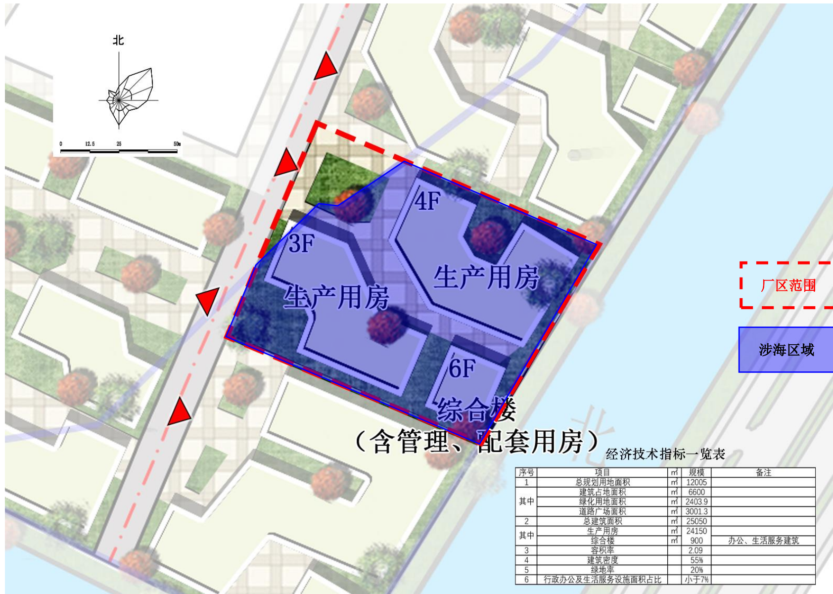
图 2.2-1 拟建高端装备项目平面布置图
