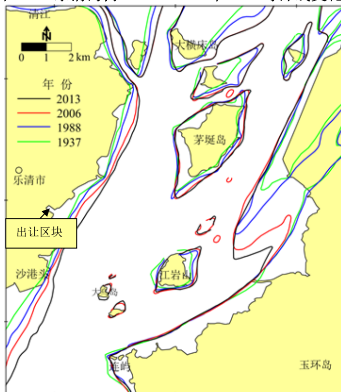
图 3.1-10 出让区块附近 1937~2013 年 0m 等深线变化图
